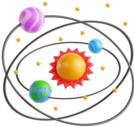
Gambar 1.1. Tata Surya Sumber: Tim ilustrator BTU 2025
